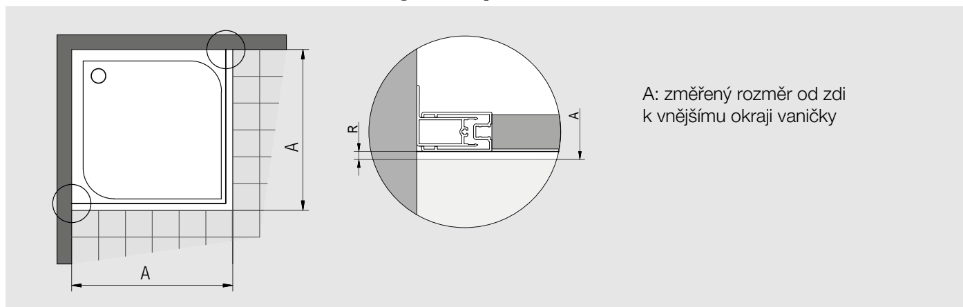
Obr. 1: Při montáži na vaničku je odsazení R (viz detail 1) závislé na velikosti rádiusu vnější hrany vaničky a je stejné pro standardní i zvláštní rozměry.
