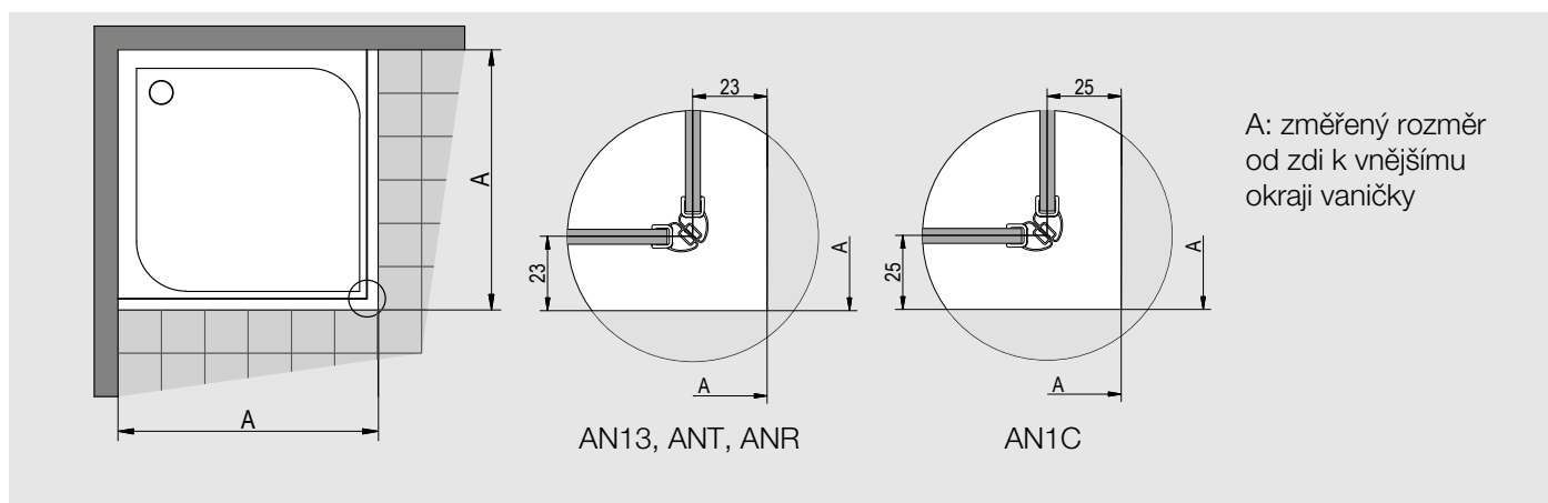
Obr. 1: Při montáži na vaničku je odsazení 23 mm (AN13, ANT, ANR), 25 mm (AN1C).
