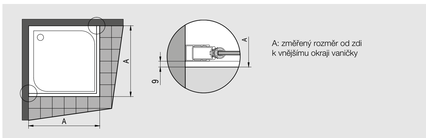
Obr. 1: Při montáži na vaničku je odsazení u všech standardních rozměrů 9 mm.
