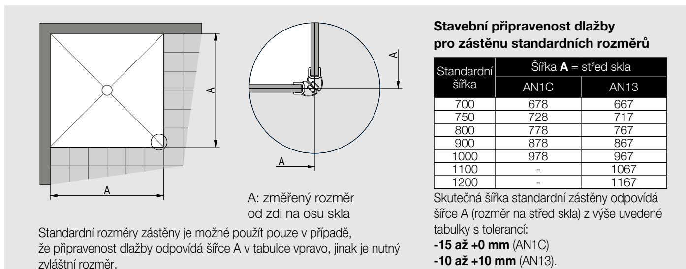
Obr. 2: U montáže na dlažbu se při výrobě nezohledňuje žádné odsazení.
