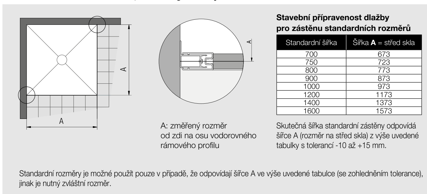
Obr. 2: U montáže na dlažbu se při výrobě nezohledňuje žádné odsazení.
